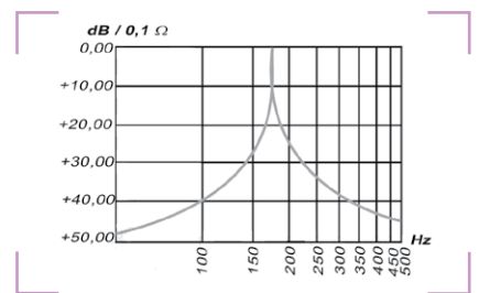
Respuesta en frecuencias típicas
